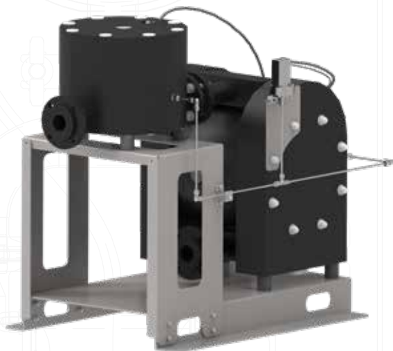
■ TXB400+DTBX400: integrované s pneumatickým systémem monitorování protřetí membrán
